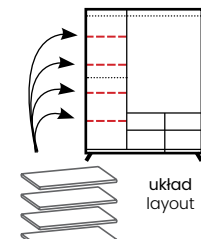
AT14 - półki do szafy AT13 (4szt) → / ↗ / ↗ 57/48/1,6
